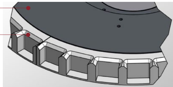
具有数个凹槽的选定槽 (3D模拟)
