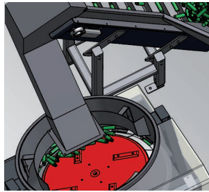
上方转盘
