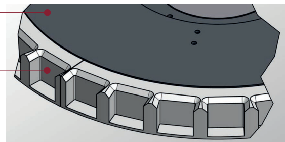
Pieza selectora con múltiples cavidades (Simulación 3D)
